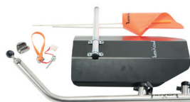
Kit fijación para bicicleta
